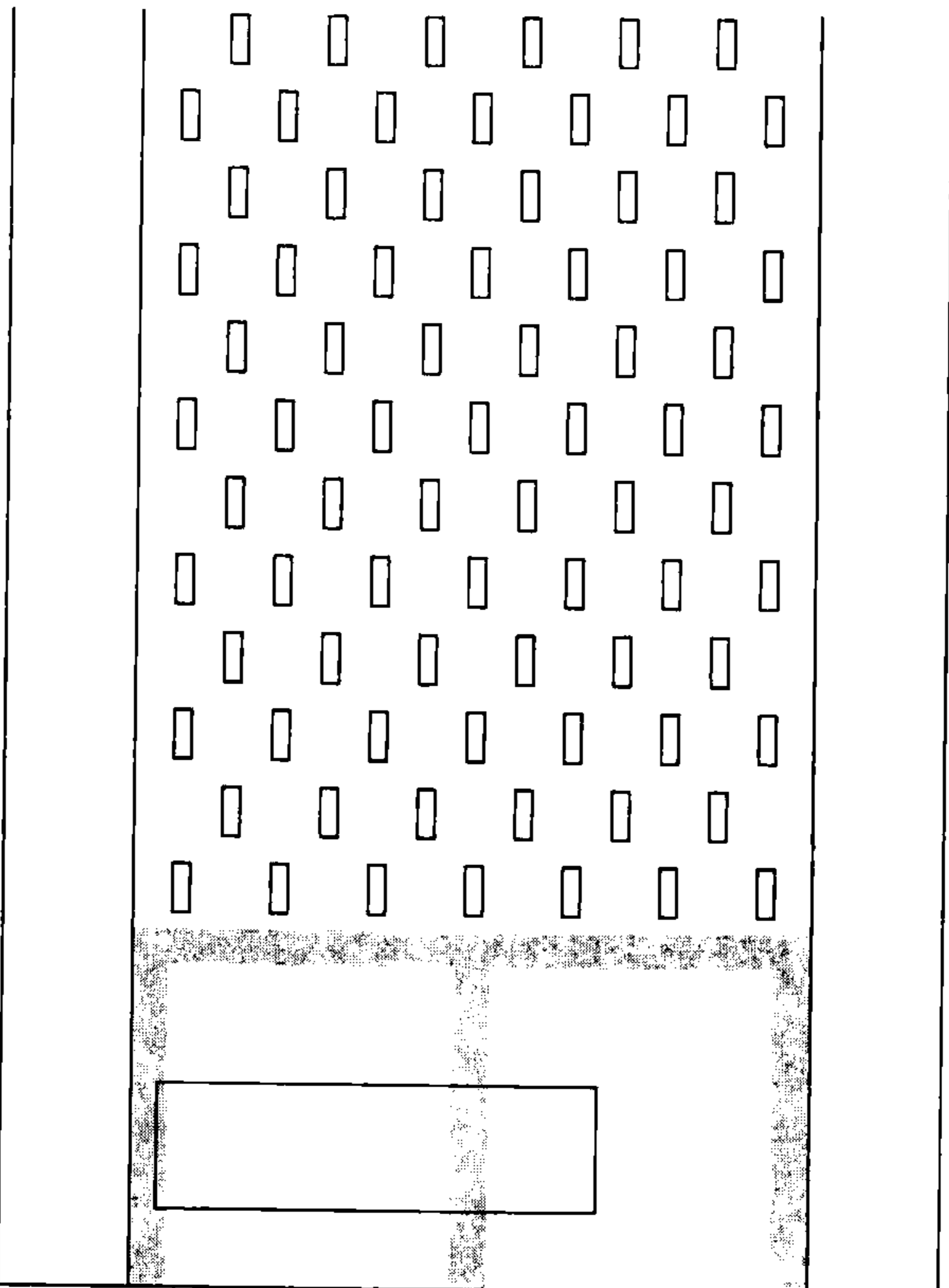
۳. نمای گرافیکی ضلع غربی مکتب نقش رستم، مقیاس یک صدم
